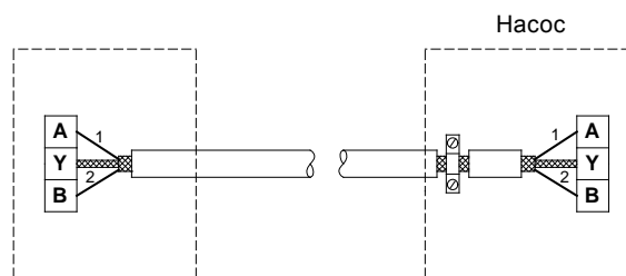
Рис. 18 Подключение 2-жильного экранированного кабеля
