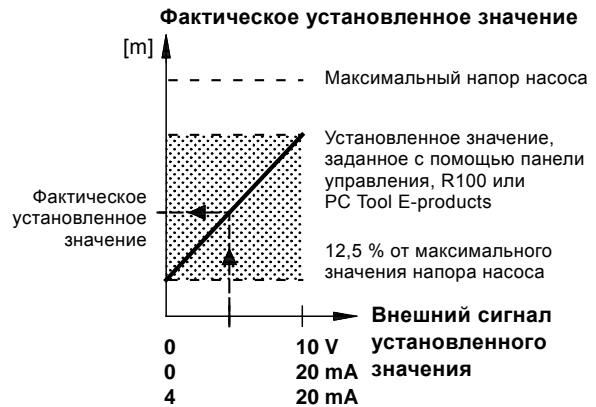
Рис. 39 Зависимость между фактическим установленным значением и внешним сигналом установленного значения при регулировании с постоянным напором
