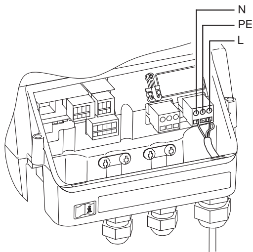
Рис. 3 Подключение электропитания
