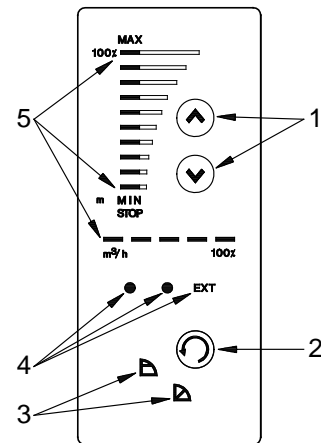
Рис. 30 Панель управления насосами с трёхфазными электродвигателями
